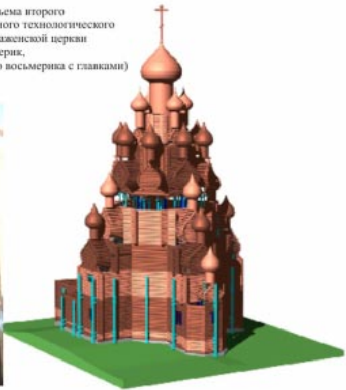
10. Макет Преображенской церкви, силовые стойки и платформы (к проекту реставрации, предложенному ЛИСИ. 1972 г.)
