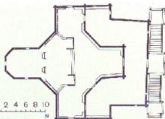
6. План Преображенской церкви (Из книги: А.В. Ополонников «русское деревянное зодчество». М., 1983. - С.274)
